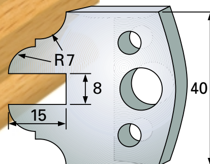
Konterprofil
