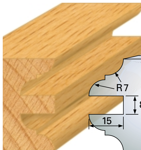
Konterprofil
