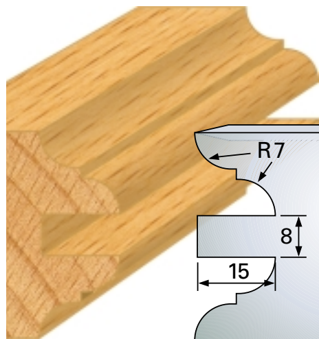
Konterprofil
